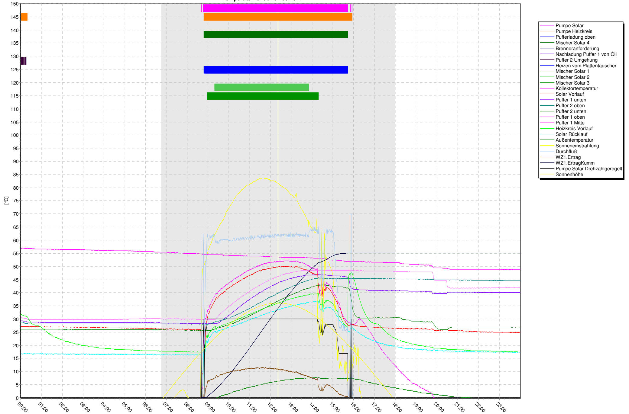
Temperaturverlauf 04.03.2011
